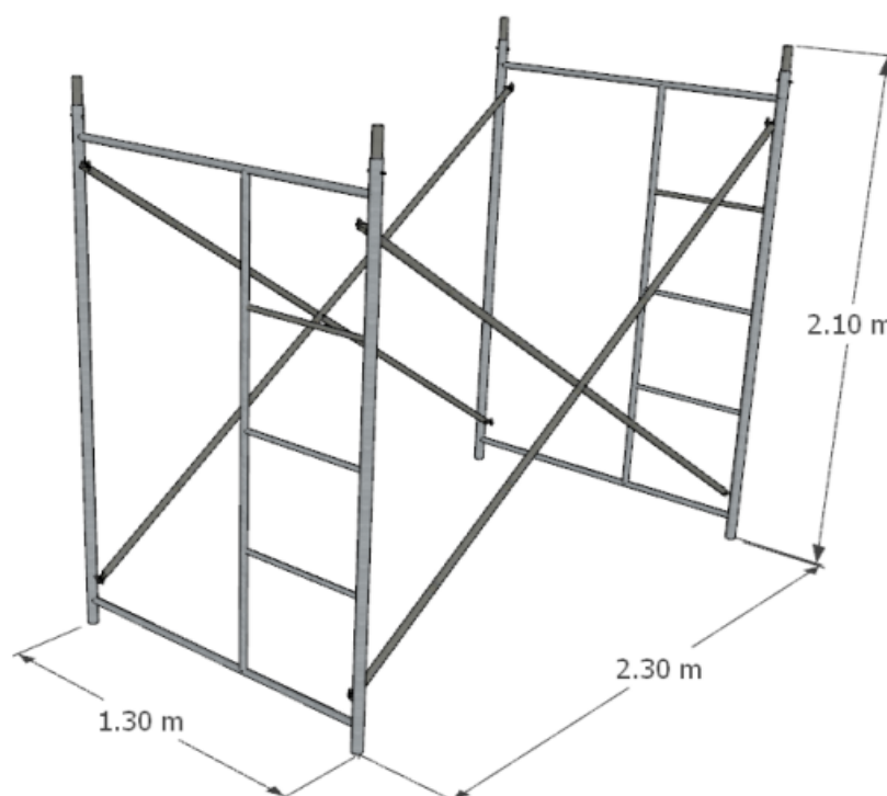
ISOMETRIA DE ANDAMIO ACROW
